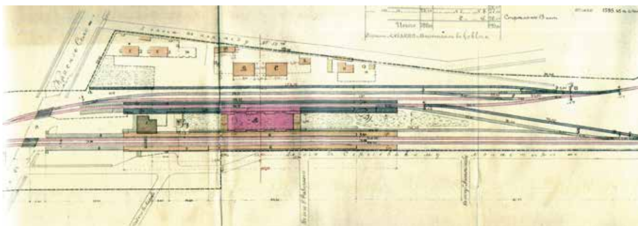
Генплан и проект станции Лигово (1890-1891)
